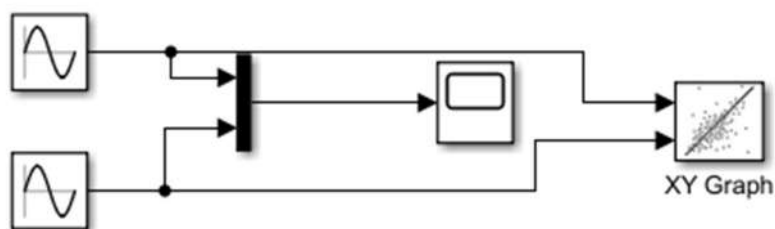
Rysunek 3 - model 3 - układ do generowania krzywych Lissajous'a
